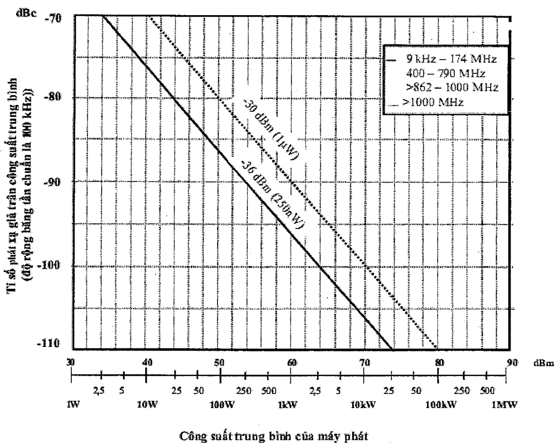
Hình 2 - Các giới hạn phát xạ giả đối với máy phát DVB-T2 (độ rộng băng tần chuẩn là 100 kHz)
