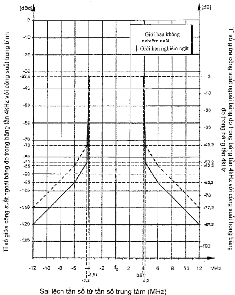
Hình 4 - Giới hạn phát xạ ngoài băng đối với các máy phát DVB-T2 có công suất từ 25 W trở lên
